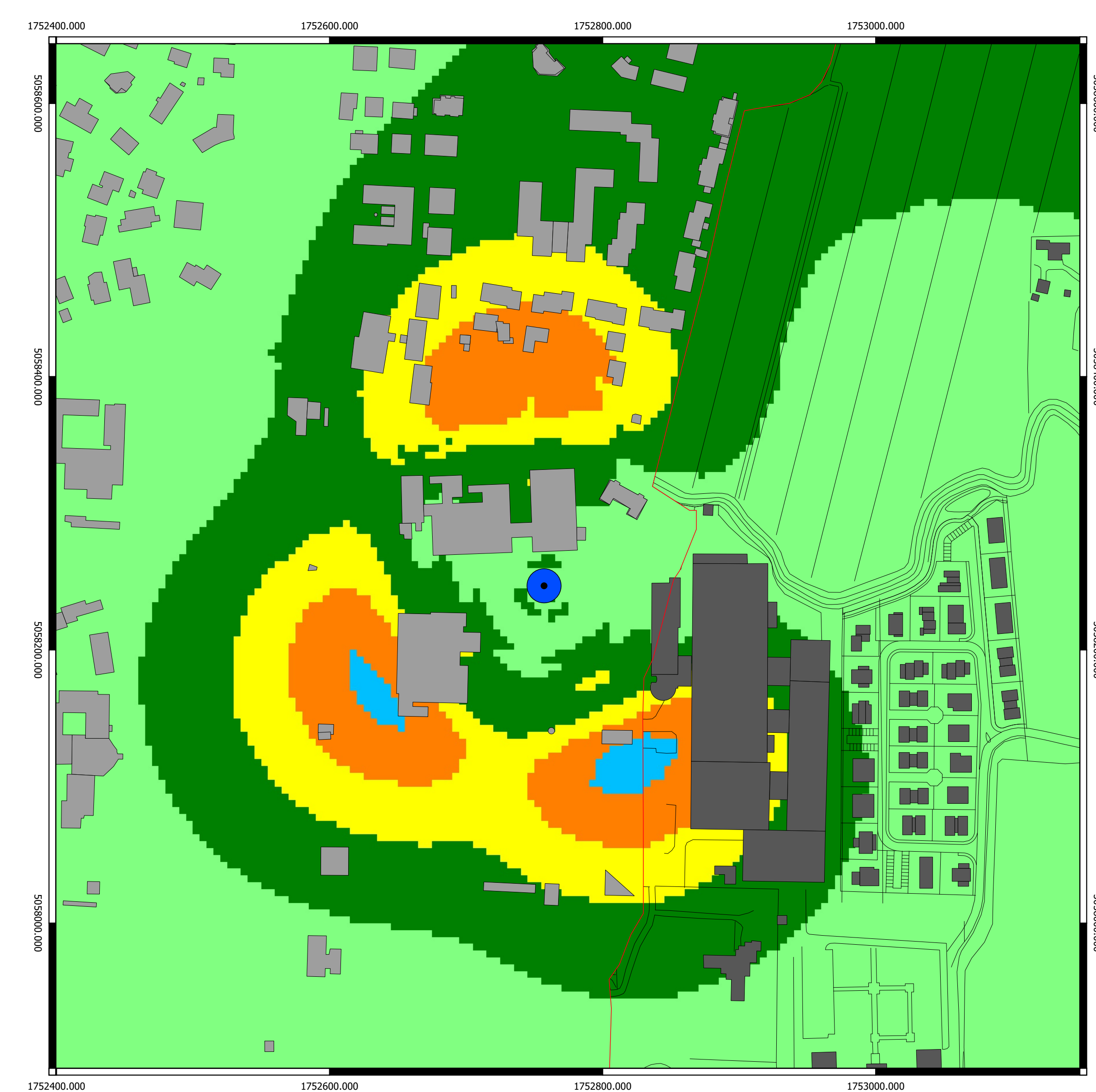
Campo elettromagnetico (V/m) calcolato alla quota di 13,3 m sul livello del terreno
