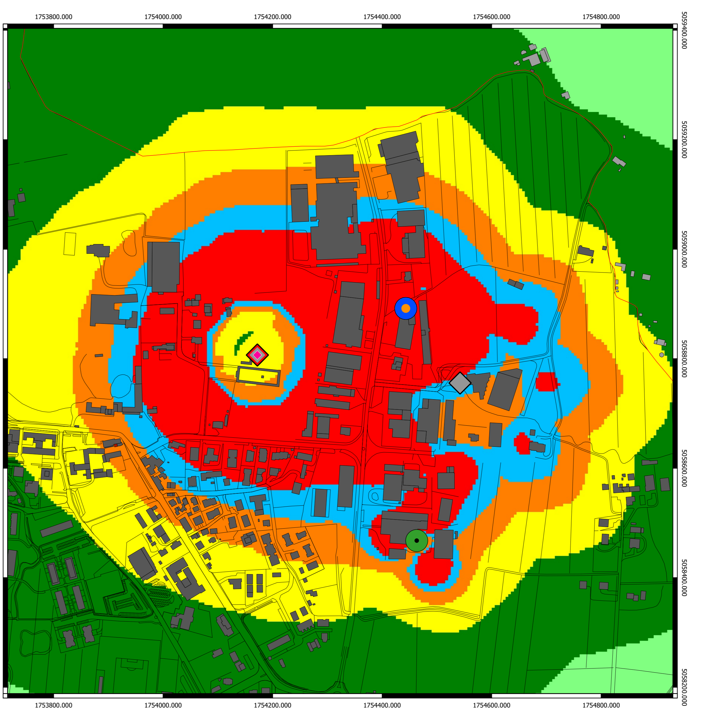
Campo elettromagnetico (V/m) calcolato alla quota di 16,4 m sul livello del terreno
